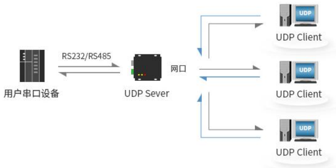
图 4-4 UDP Server
