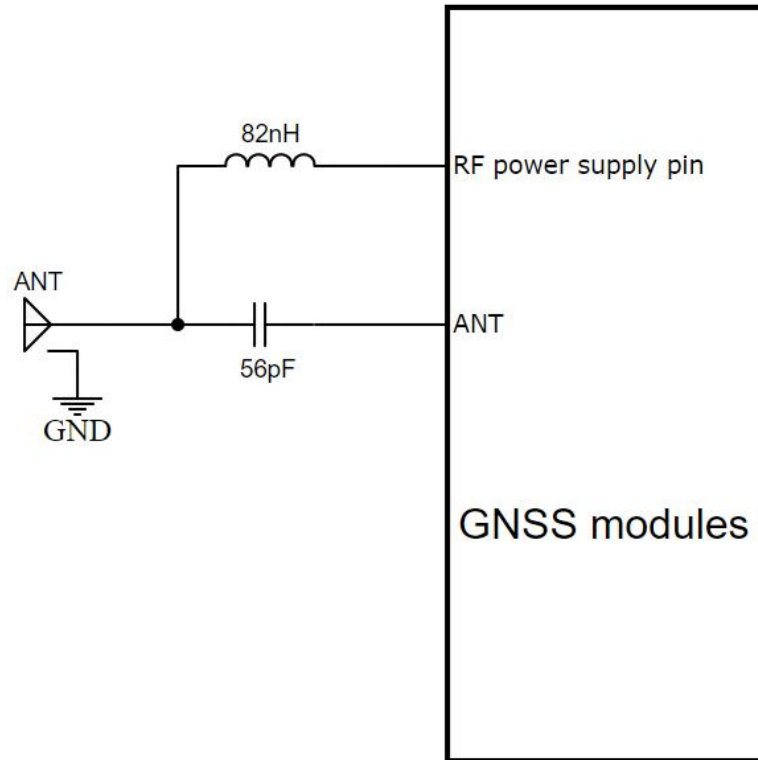
有源天线推荐接线图
