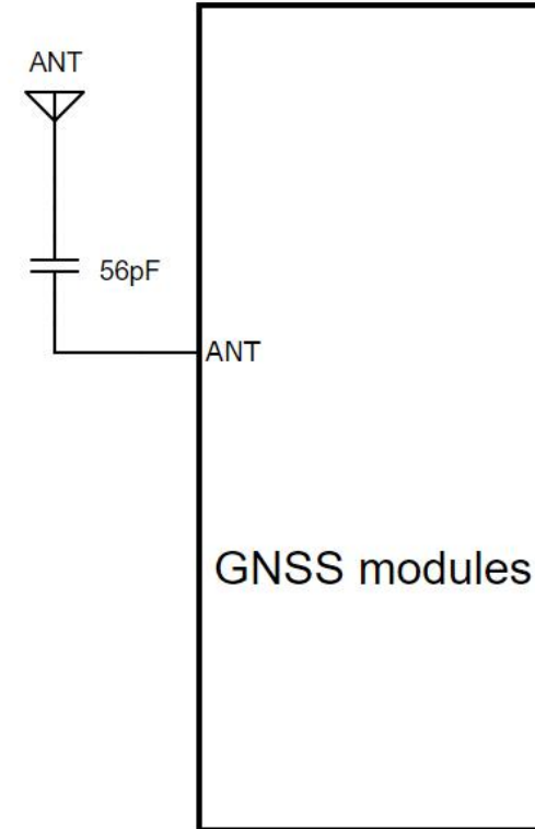
无源天线推荐接线图
