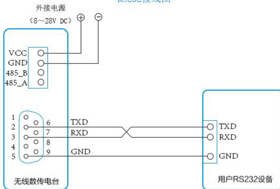
RS232接线图
