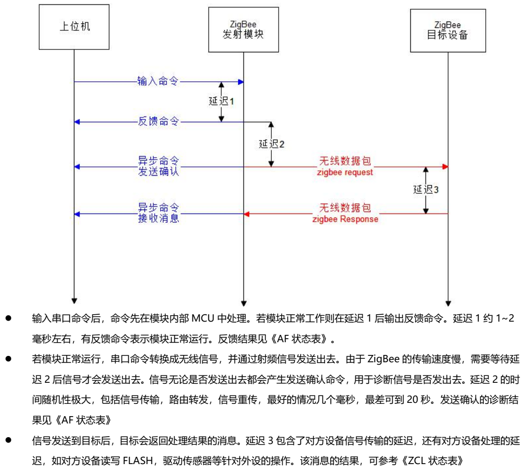
串口命令的三层返回示意图
