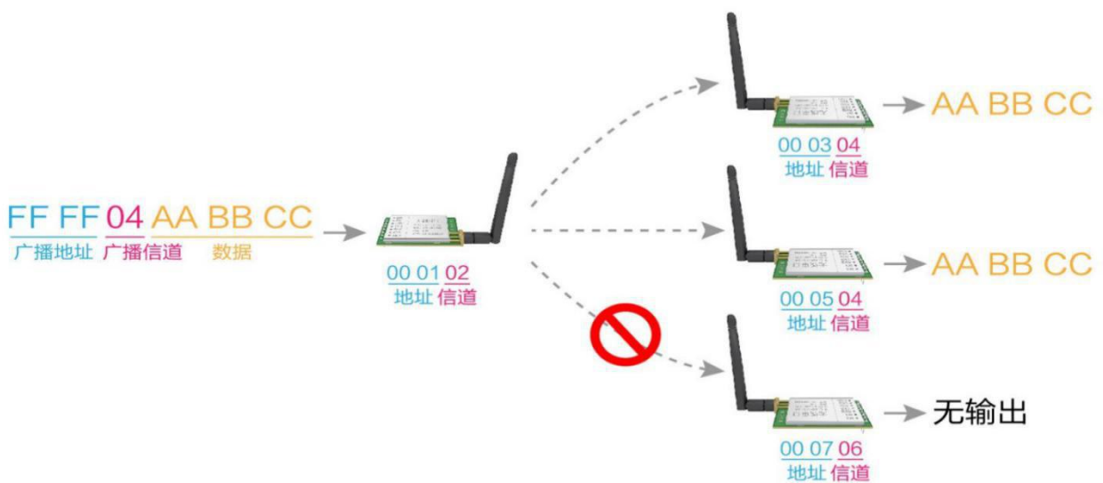
图 5-2 广播发射
