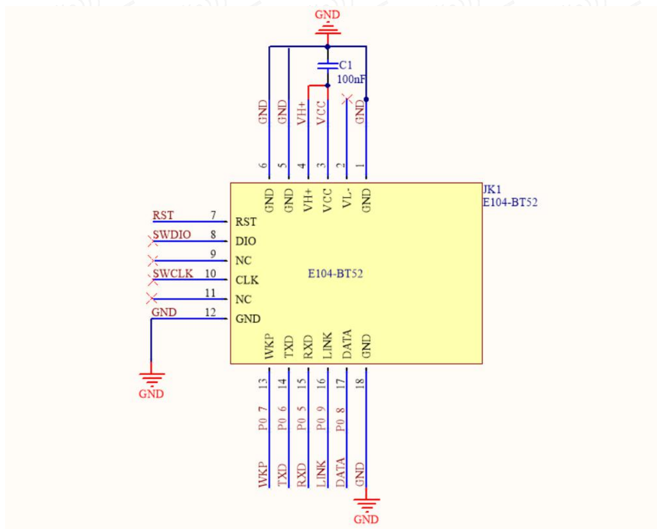
图 5-1 电路
