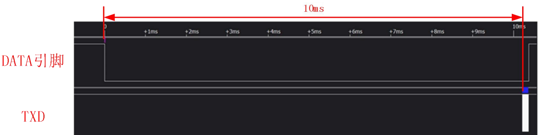
图表 五- 7 数据输出延迟图
