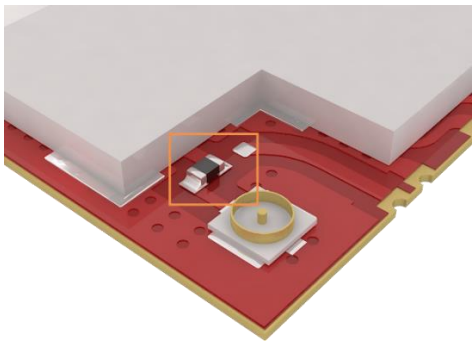
使能 IPEX 接口（默认）
